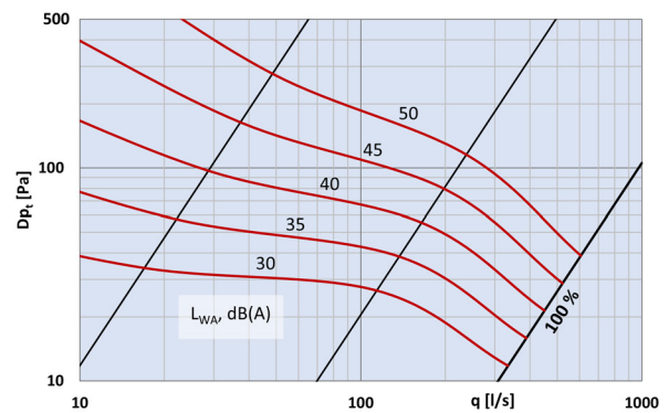
Diagram 6: Total A-vägd ljudefektnivå, dB(A) för SPMF-315
