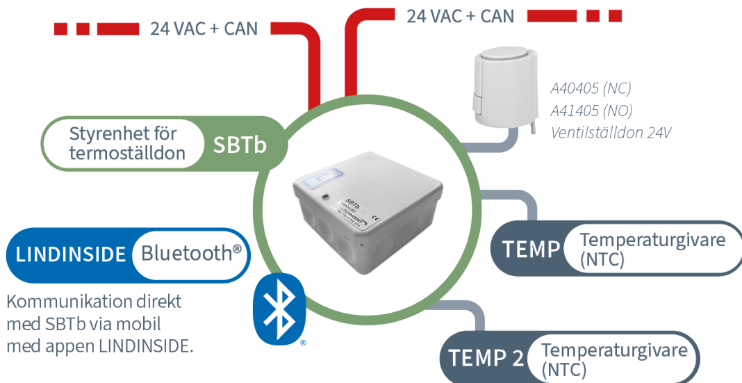
Anslutningsschema för SBTb.
