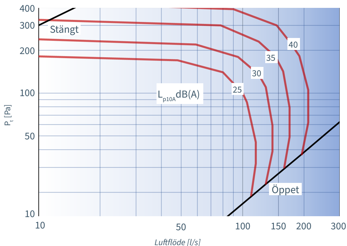
Diagram ISQ-FM, Ljudtrycksnivå L_{p10A} dB(A)
