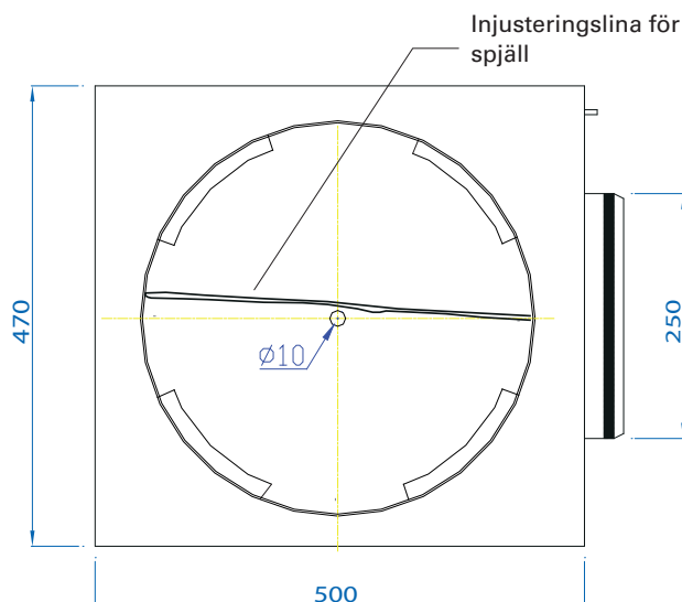
MTK: Vy underifrån. Mått i mm.
