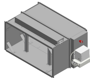
DCV-CF rektangulär: Regulator CFL och spjällmotor monterade på ett rektangulärt spjäll med en anslutande mätfläns.
