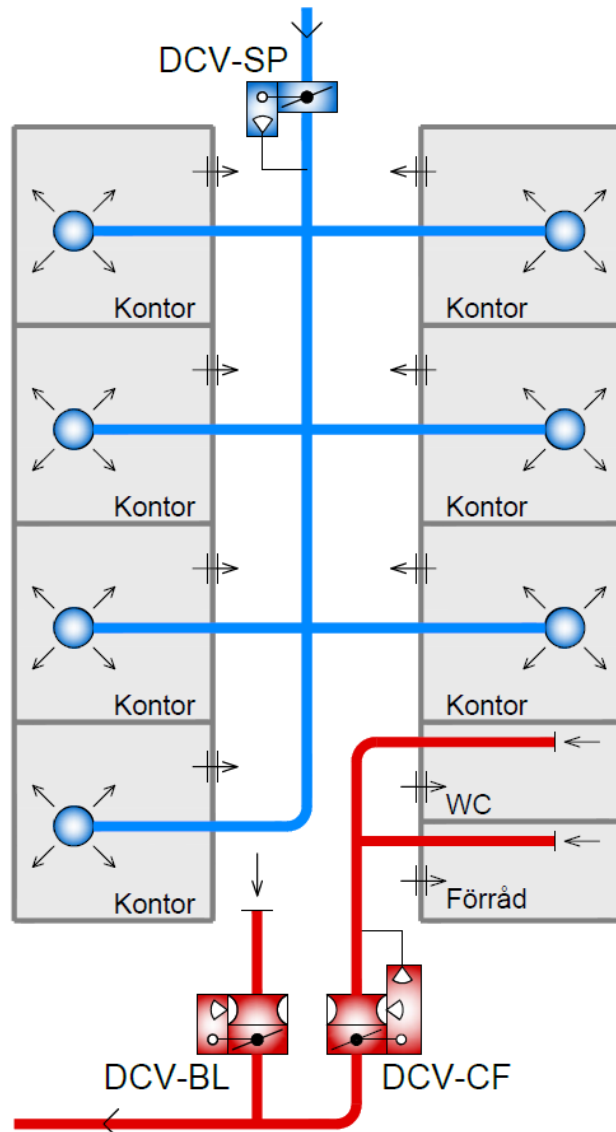
Exempel på funktionsschema med DCV-CF: Kontorslösning.
