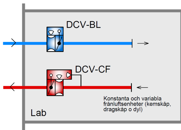
Exempel på funktionsschema med DCV-CF: Laboratorie.
