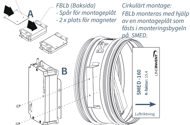
Illustration 1M. Montage av FBLb på mätfläns.
