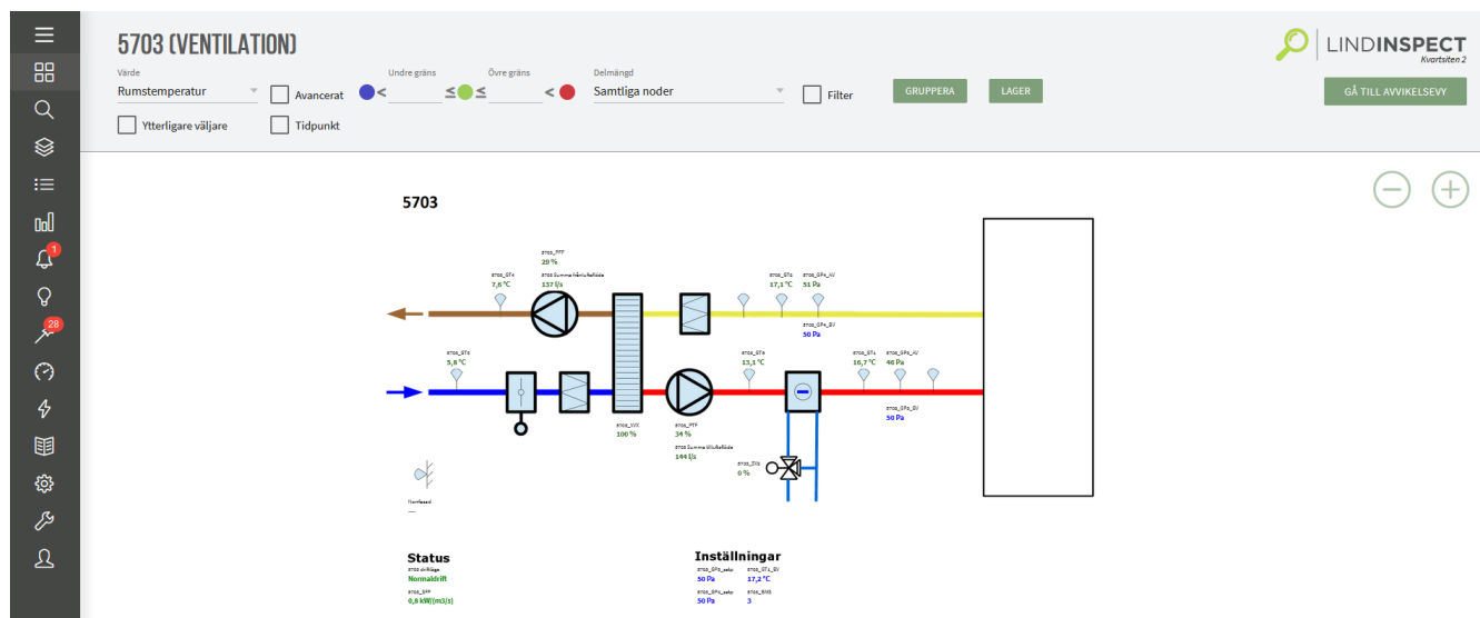
Visualisering af ventilationsaggregat i LINDINSPECT®.
